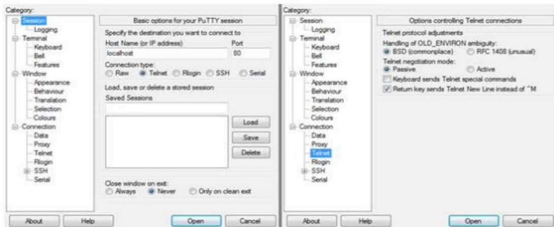
Rysunek 2 - Ustawienia Putty
